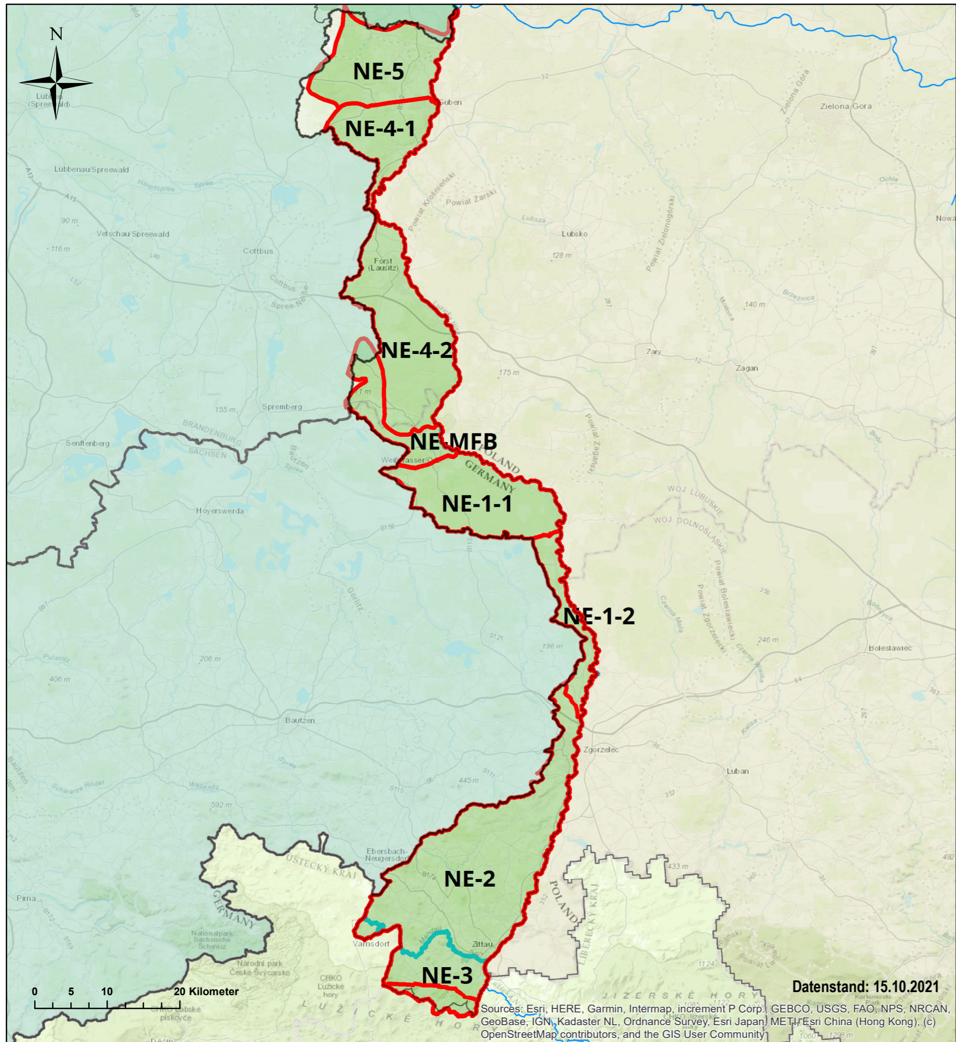
BG LAN - Karte 13.2 - Chemischer Zustand der Grundwasserkörper hinsichtlich Nitrat - Vergleich 2. und 3. Bewirtschaftungszeitraum
