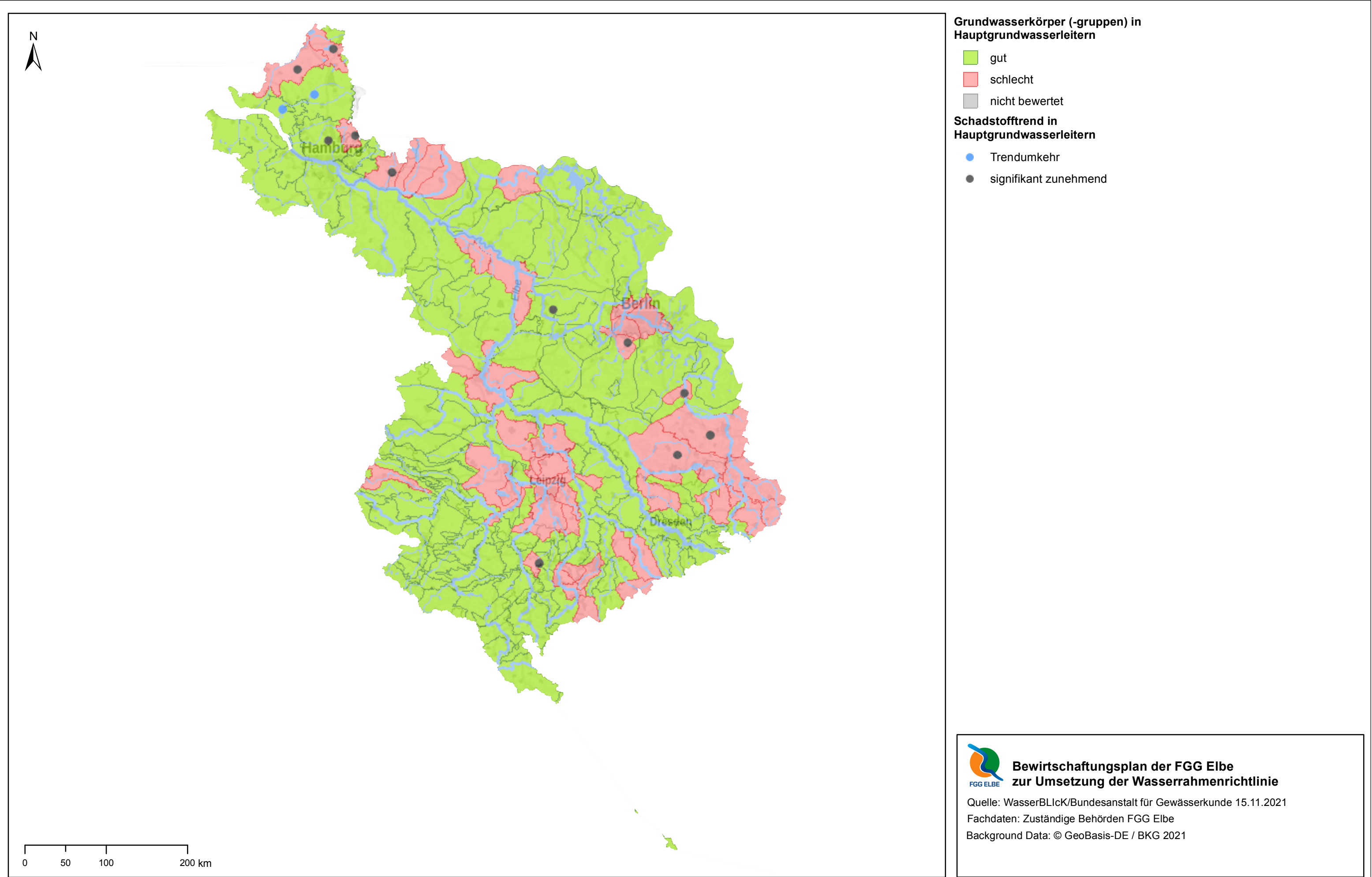
FGG Elbe - Karte 4.7.3: Chemischer Zustand der Grundwasserkörper hinsichtlich Schadstoffen nach Anhang II der Tochterrichtlinie Grundwasser und anderen Schadstoffen (inkl. nicht relevanter Metaboliten)
