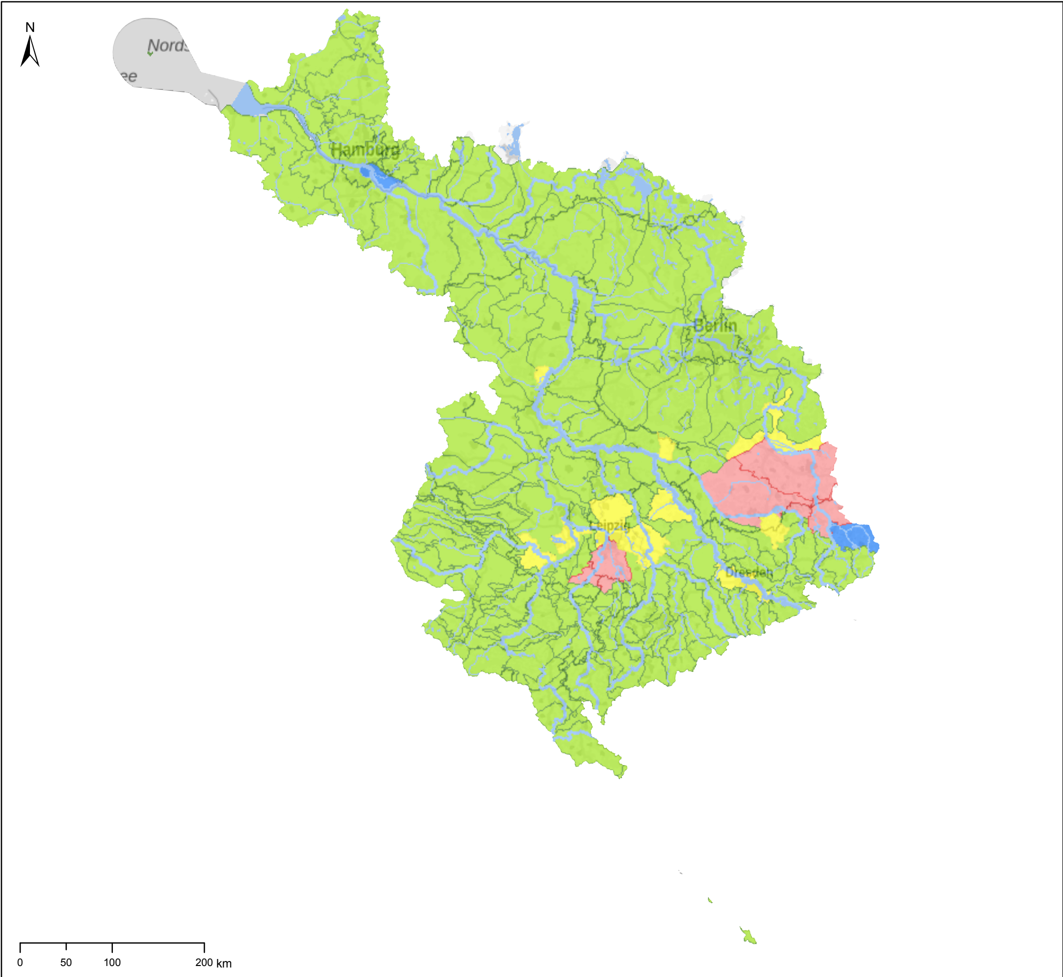
FGG Elbe - Karte 13.3: Mengenmäßiger Zustand der Grundwasserkörper in Hauptgrundwasserleitern - Vergleich der Ergebnisse für den 2. und 3. Bewirtschaftungszeitraum
