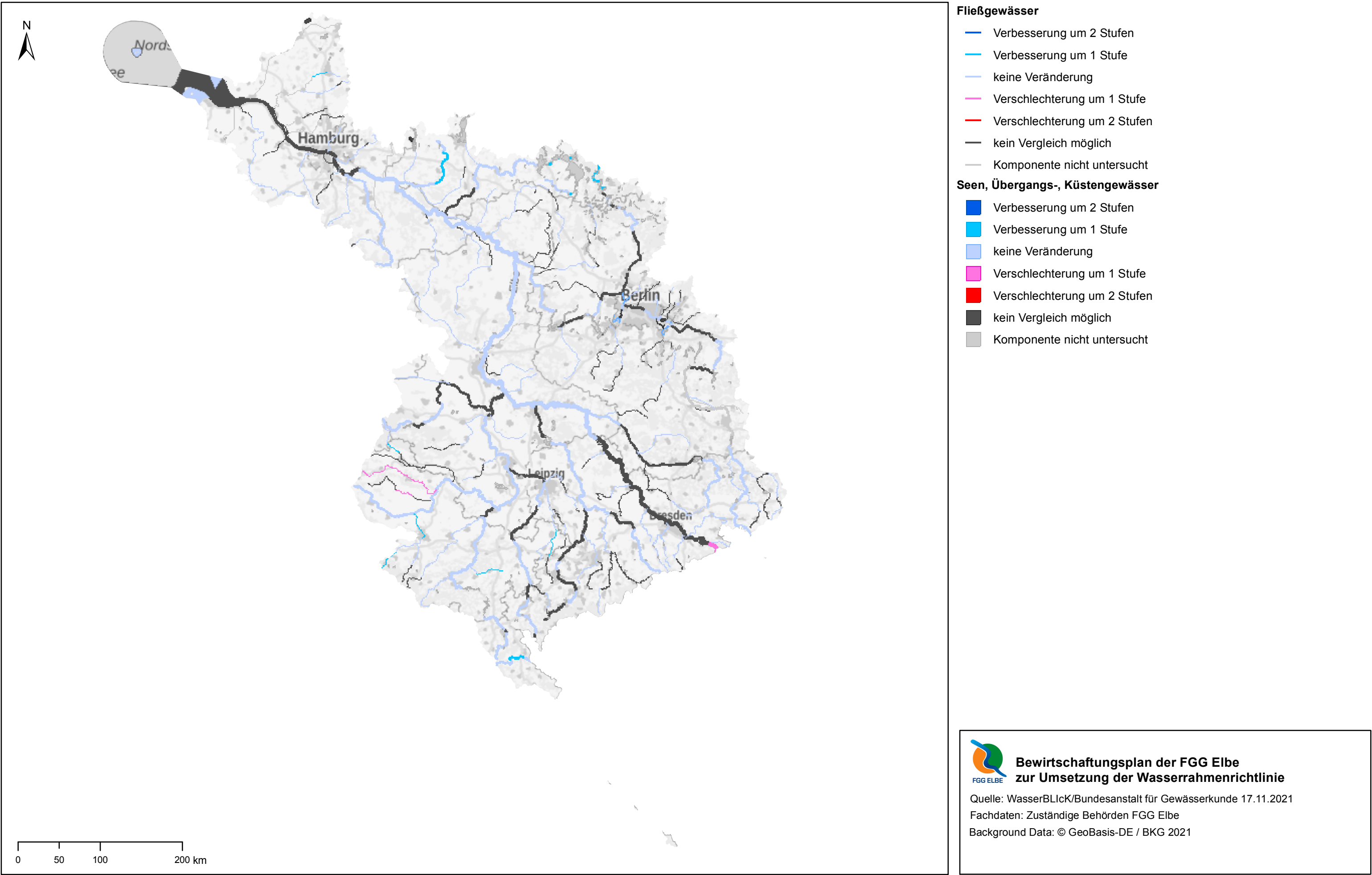
FGG Elbe - Karte 13.1.3: Ökologischer Zustand der Oberflächenwasserkörper: Vergleich der Überwachungsergebnisse der Qualitätskomponente Makrozoobenthos für den 2. und 3. Bewirtschaftungszeitraum
