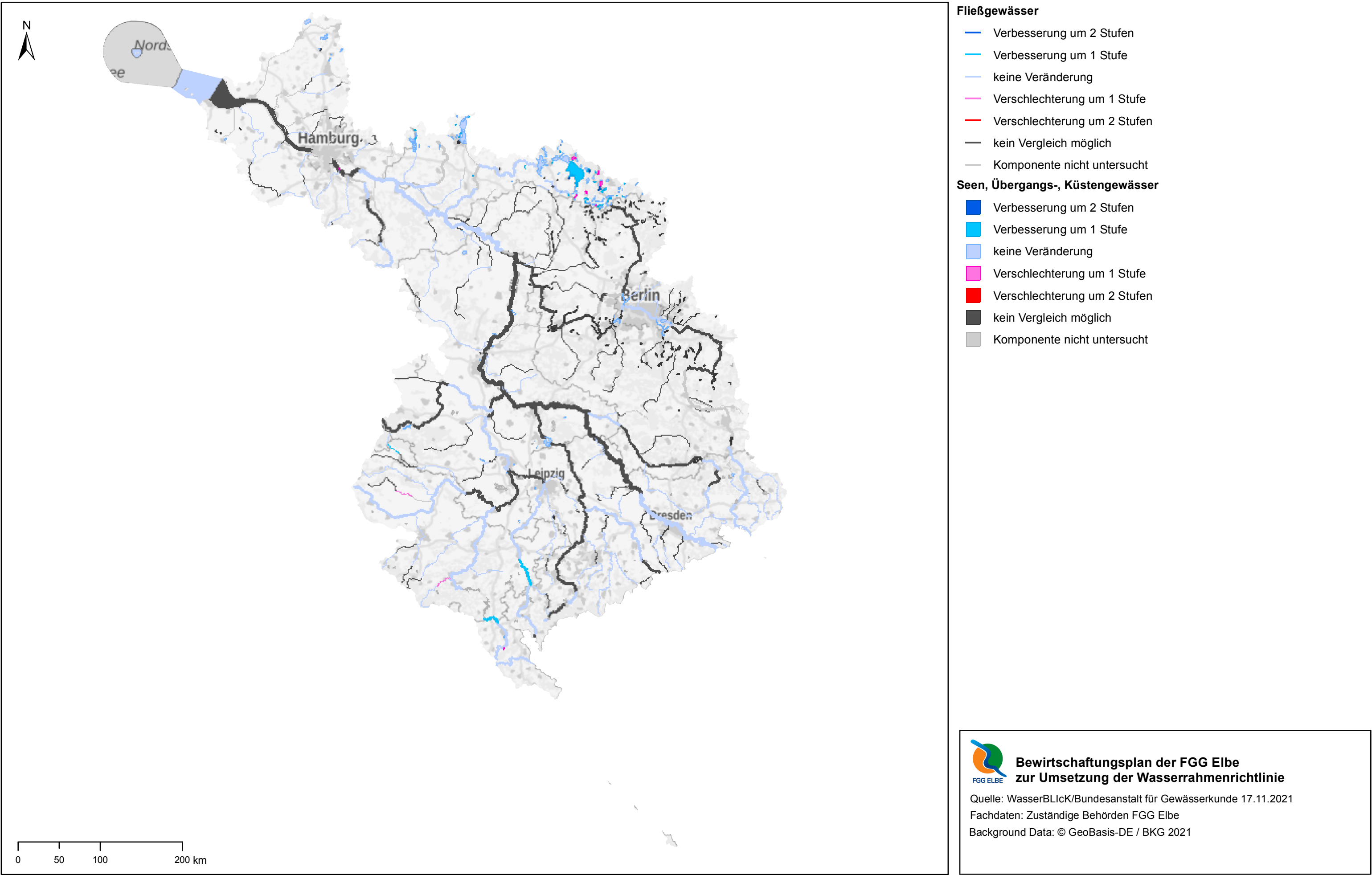
FGG Elbe - Karte 13.1.2: Ökologischer Zustand der Oberflächenwasserkörper: Vergleich der Überwachungsergebnisse der Qualitätskomponente Makrophyten/Phytobenthos für den 2. und 3. Bewirtschaftungszeitraum
