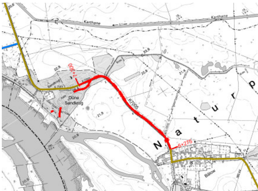
Lageplan
