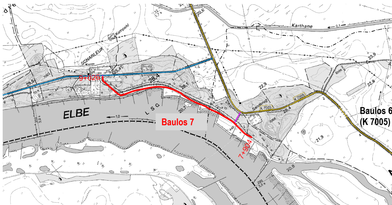
Lageplan
