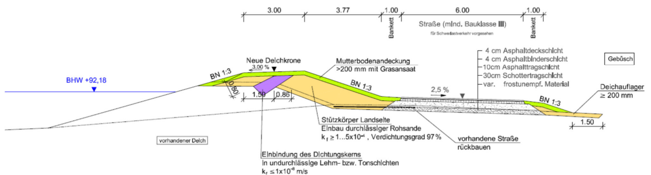
Abb. 2: Darstellung Regelprofil BA 3.3.2
